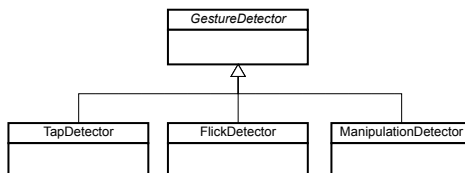
Figur 3.2. UML-diagram som visar subclasserna till GestureDetector .
