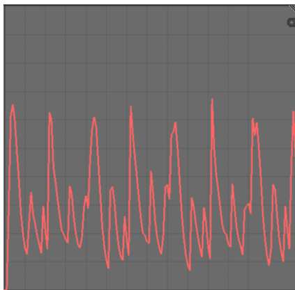
Figur 3.6 Illustration av ljudvågor,
