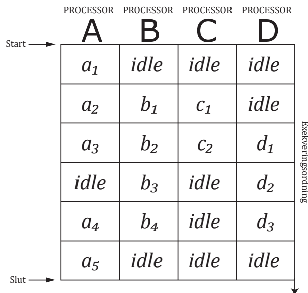
Figur 2.1. Exempel på en synkon, parallell algoritm fördelad på fyra processorer med någon specifik input.
