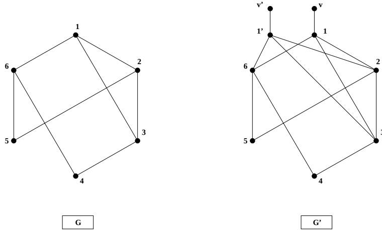
Figur 1: En graf G och hamiltonstigsreduktionens konstruerade graf G' .
